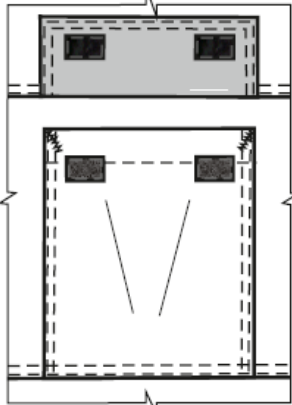
Нагрудный карман полукомбинезона для ИТР
