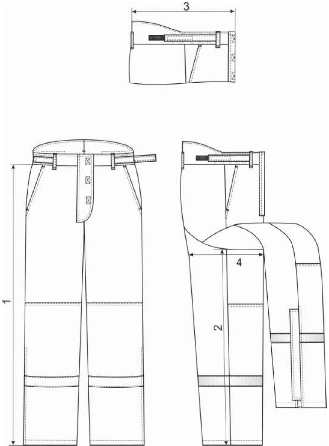
Рисунок 10 – Схема измерений брюк
