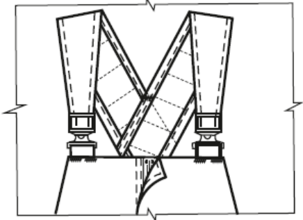
Застежка бретелей полукомбинезона
